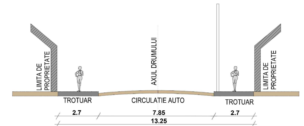
PROFIL STRADAL TRANSVERSAL STR.FURNICILOR
